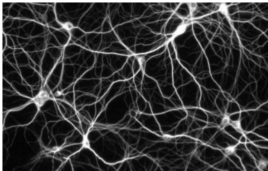
Abbildung: Neuronennetz
